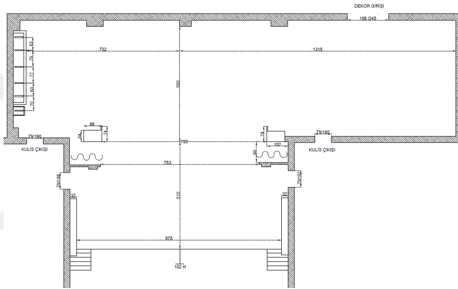
Şekil 91: Altındağ Tiyatrosu Sahne Planı [URL 9]
