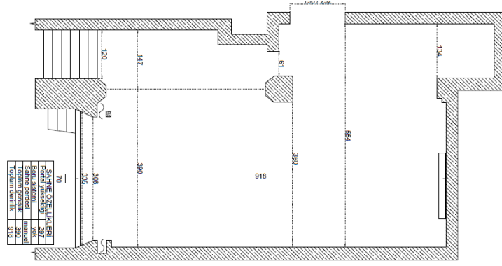
Şekil 74: Oda Tiyatrosu Sahne Plan [URL 9]
