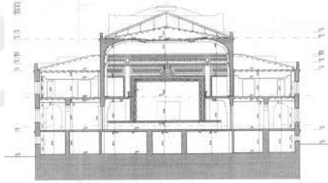
Şekil 56: Türk Ocağı Merkez Binası Kesit (Bozdağ 2013:179)
