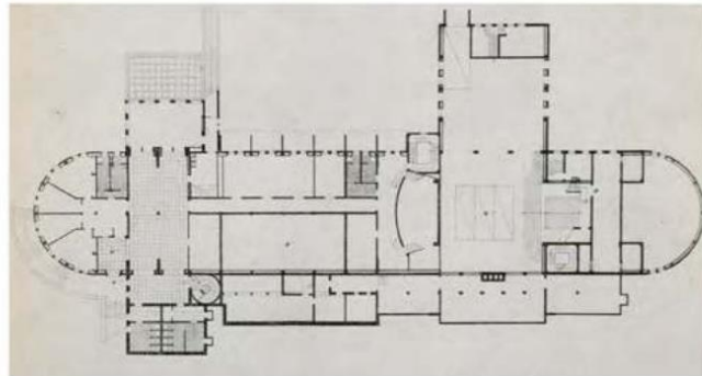
Şekil 82: Sergi evi – Opera binası bodrum kat karşılaştırma (Pekdemir 2021:96)
